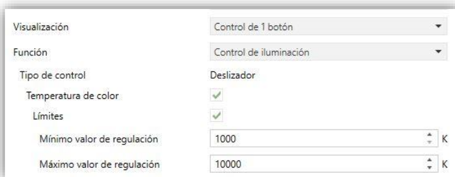
Figura 56. Control de 1 botón - Control de iluminación
