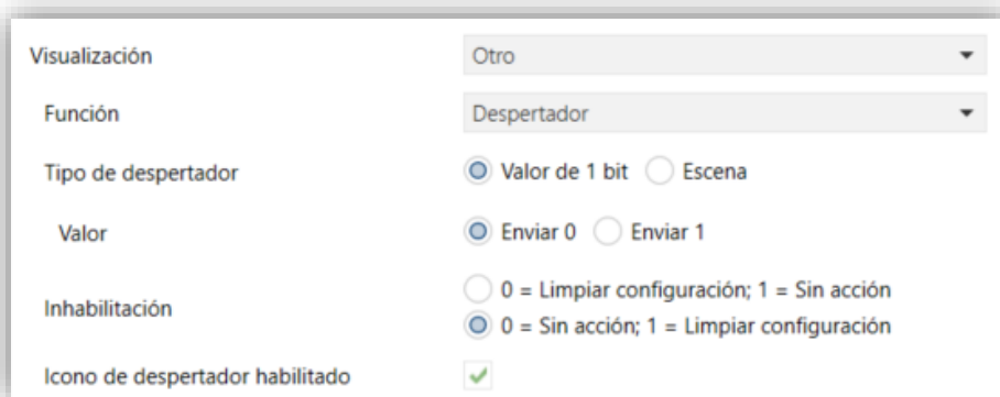
Figura 87. Despertador
