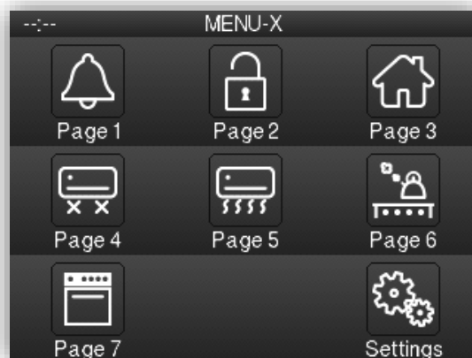
Figura 20. Menú.
