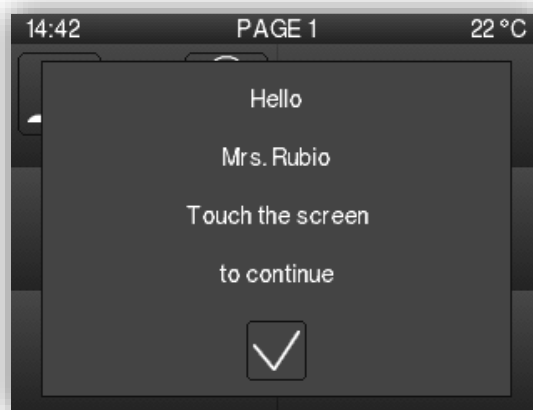
Figura 17. Mensaje emergente
