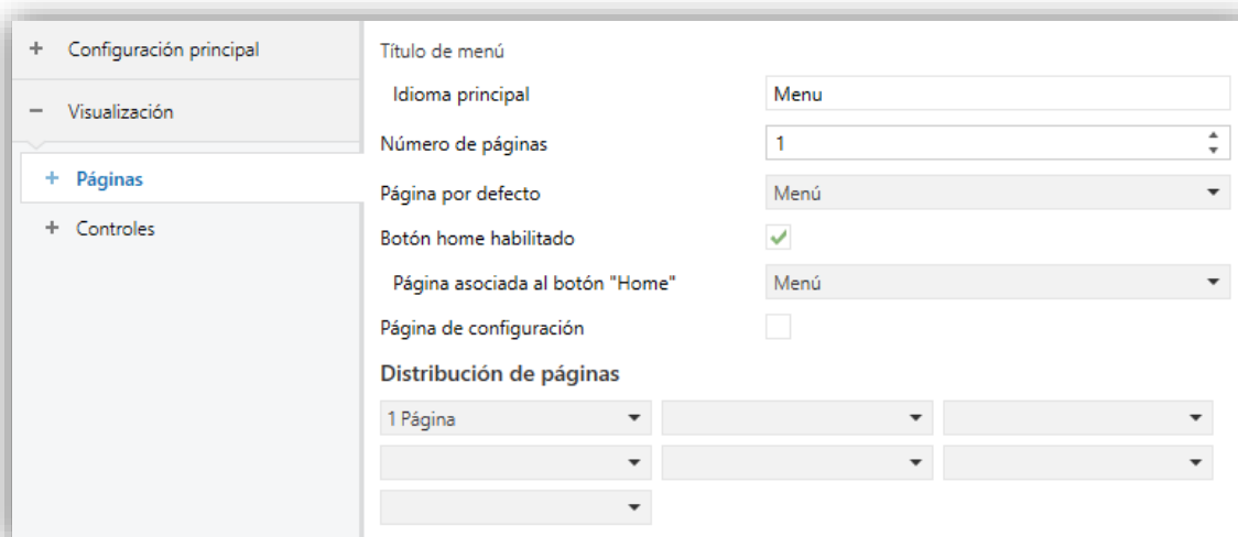
Figura 27. Páginas - Configuración.
