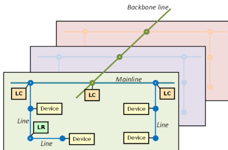
Figura 1 Contexto (topología)
