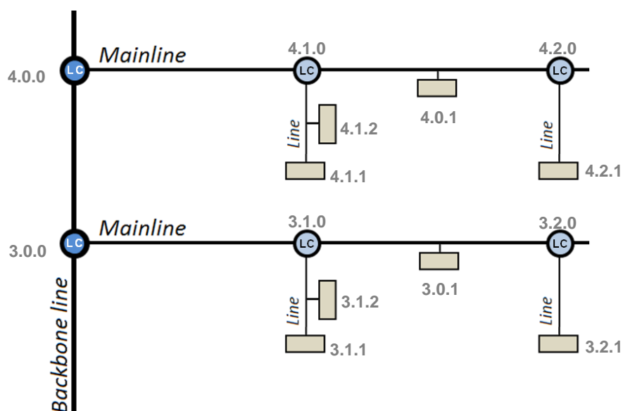
Figura 3 Acoplamiento de líneas
