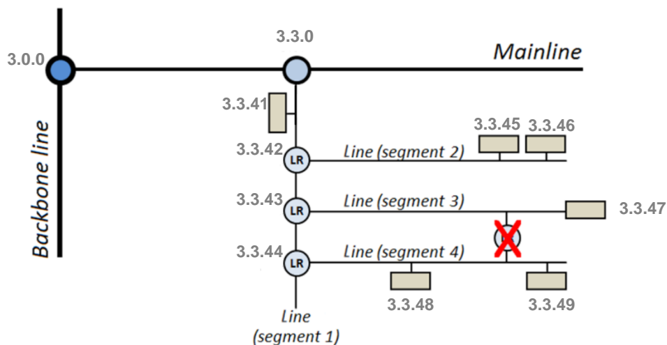
Figura 6 Situación no permitida: segmentos con dos conexiones al bus
