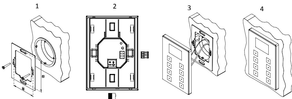
Figura 2 Instalación del TMD-Display One.
