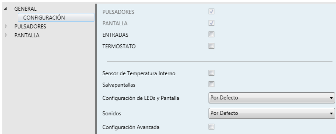
Figura 5 General - Configuración.
