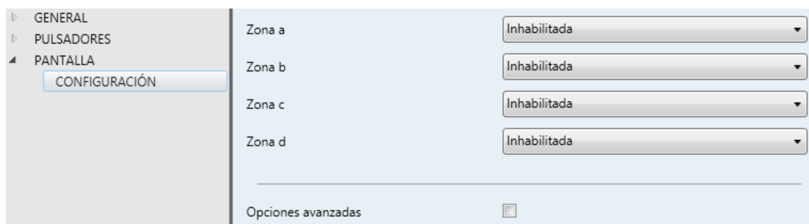
Figura 55 Pantalla - Configuración.
