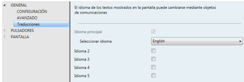
Figura 14 General - Traducciones.
