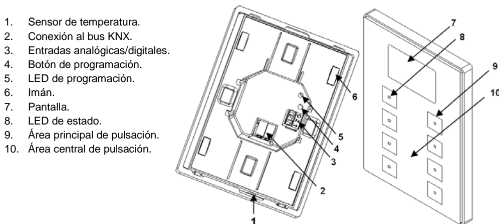
Figura 3 Esquema de elementos.
