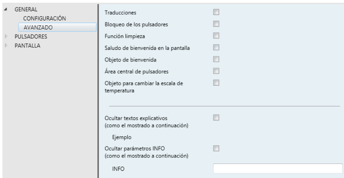
Figura 11 General - Avanzado.
