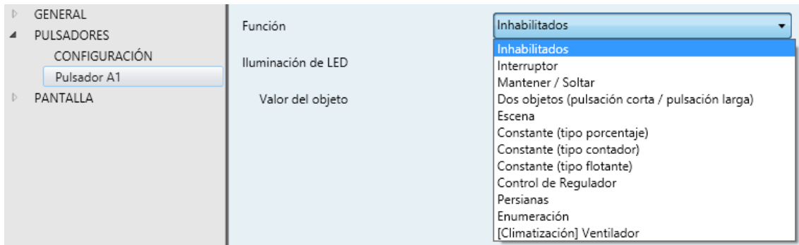
Figura 43. Pulsador individual.
