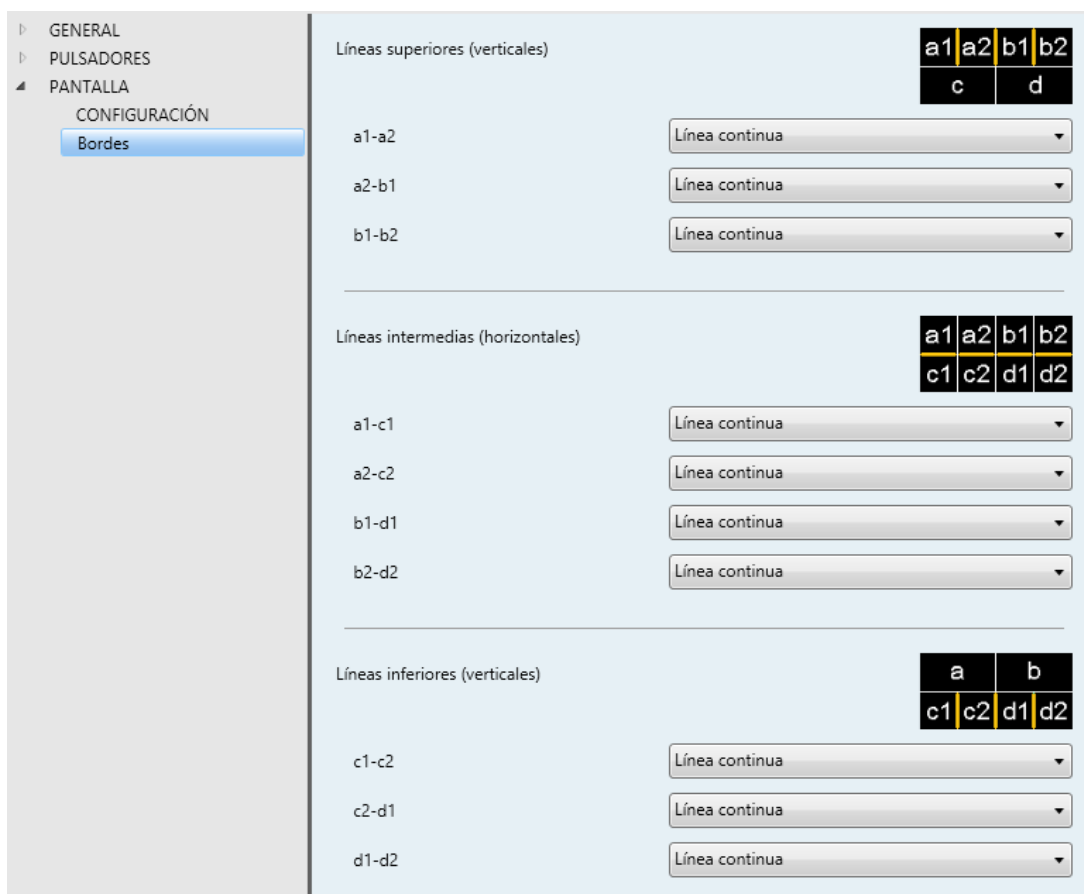
Figura 72 Pantalla - Bordes.
