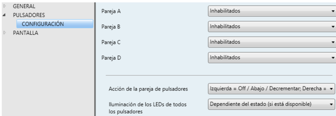
Figura 25 Pulsadores - Configuración.
