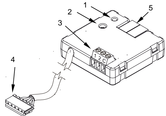
Figura 1: KLIC-DD v3
