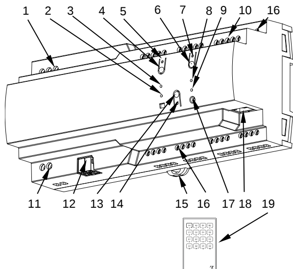
Figura 1: ALLinBOX 1612 v2
