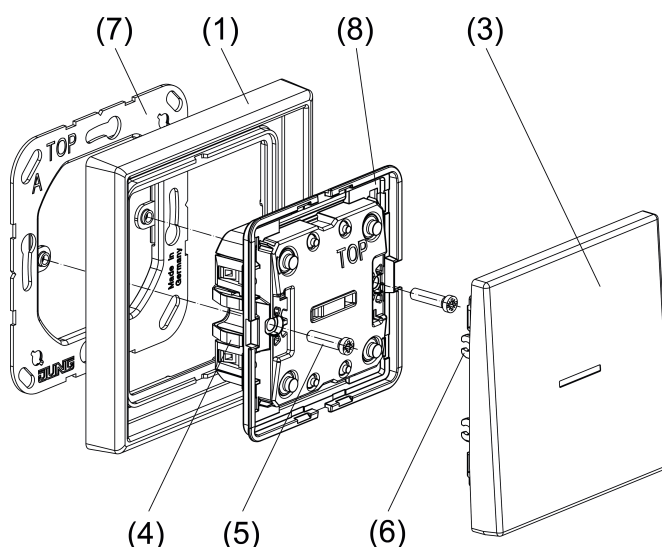
Figura 3: Montar el aparato
