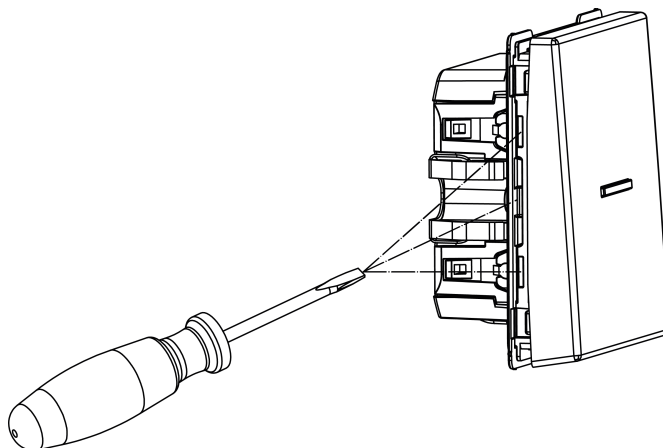
Figura 7: Desmontaje del interruptor basculante, vista lateral
