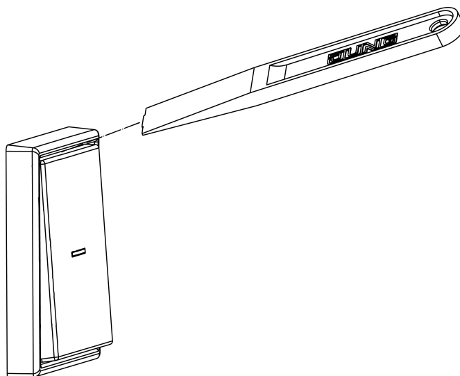
Figura 8: Desmontaje del interruptor basculante, vista superior
