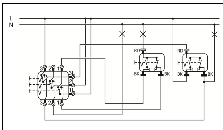
Ejemplo de conexionado 5306 EU
