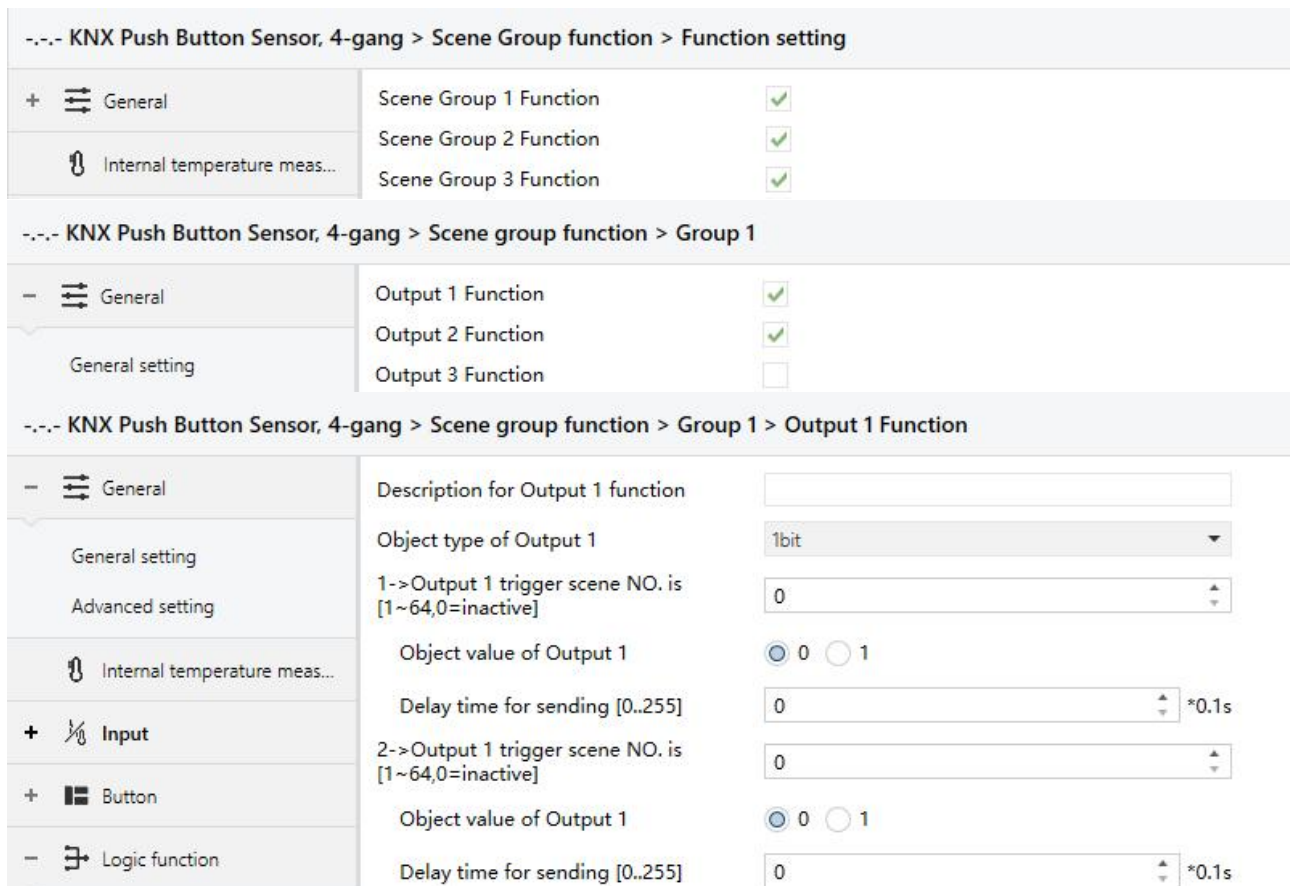
Fig.5.6 "Scene Group" parameter window
