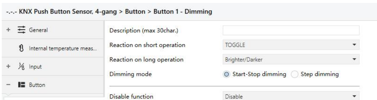
Fig.5.4.2 Parameter setting of dimming function
