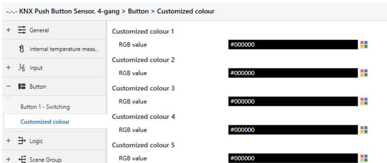
Fig.5.4.15 “Customized colour” parameter window
