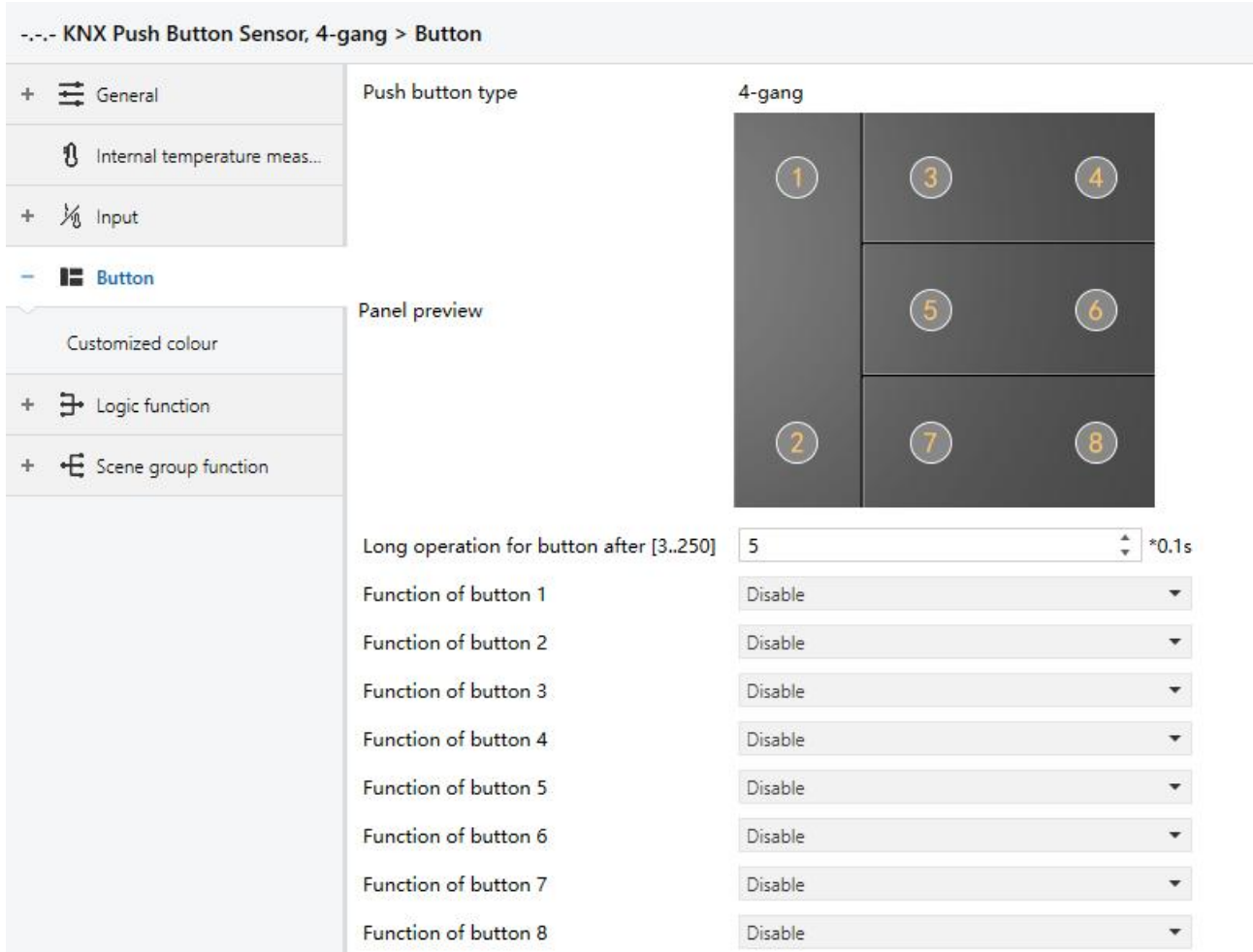
Fig.5.4 “Button” parameter window
