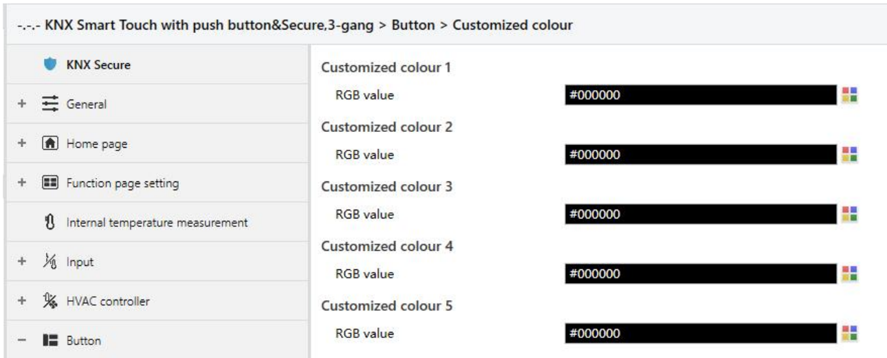
Fig.5.8.3 “Customized colour” parameter window
