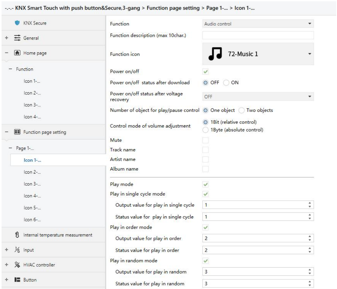
Fig.5.7.2.5 Audio control function parameter window
