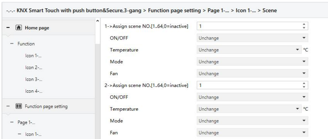
Fig.5.7.2.2(4) Air condition-Scene parameter window
