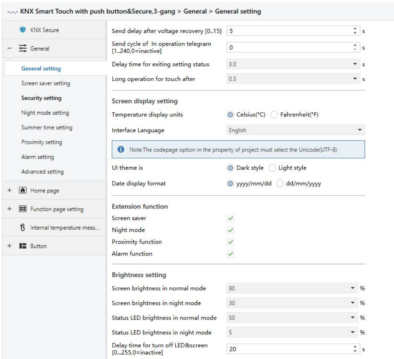
Fig.5.2.1 “General setting” parameter window
