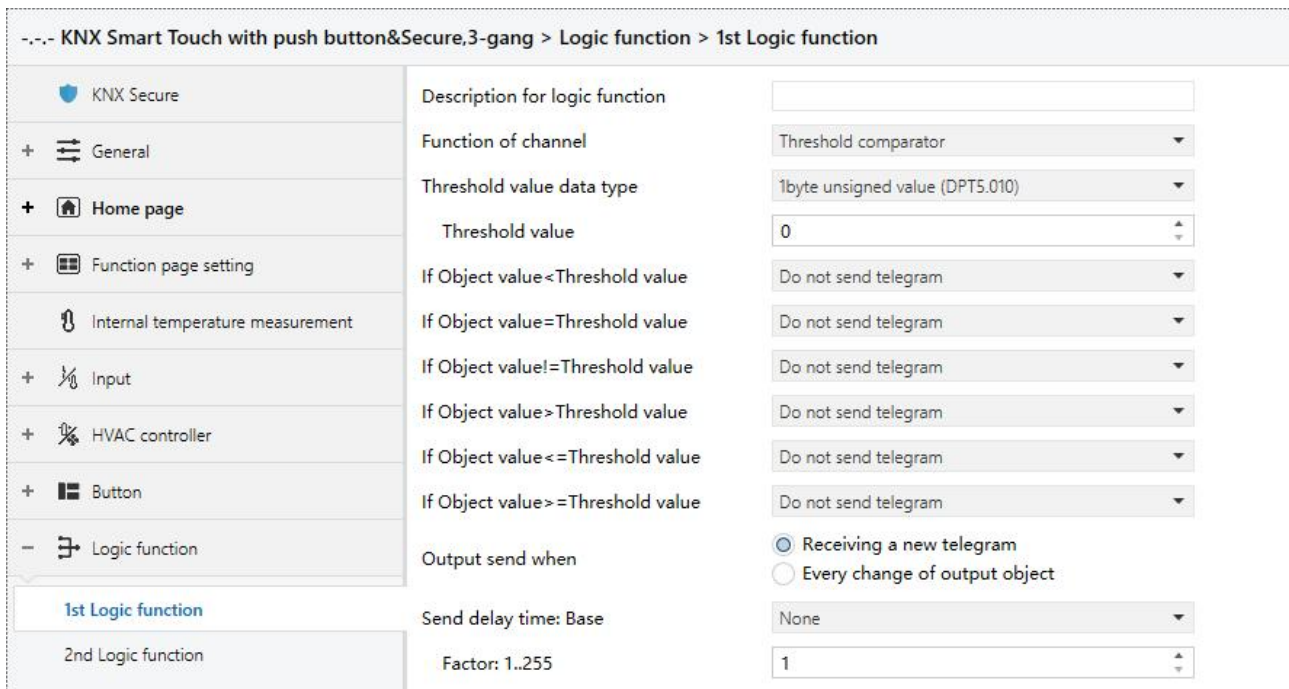
Fig.5.9.3 “Threshold comparator” parameter window
