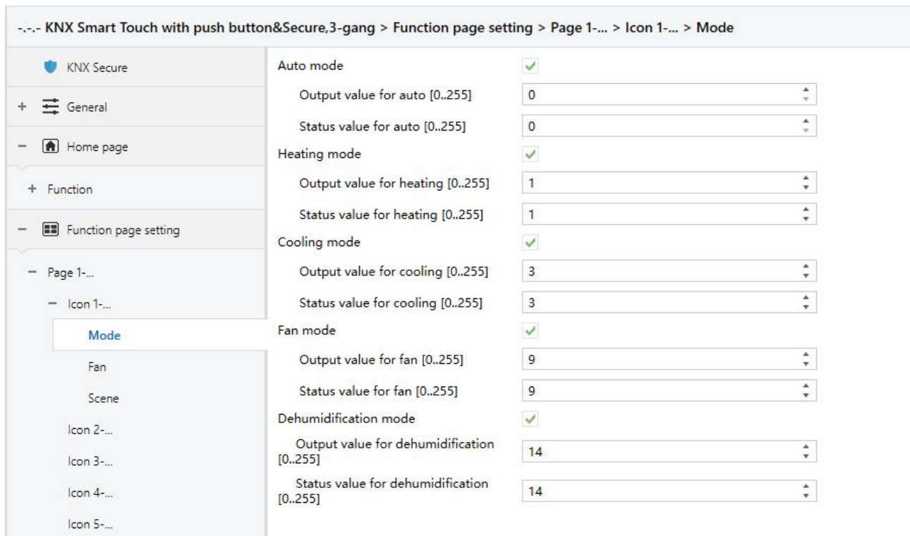
Fig.5.7.2.2(2) Air condition-Mode parameter window
