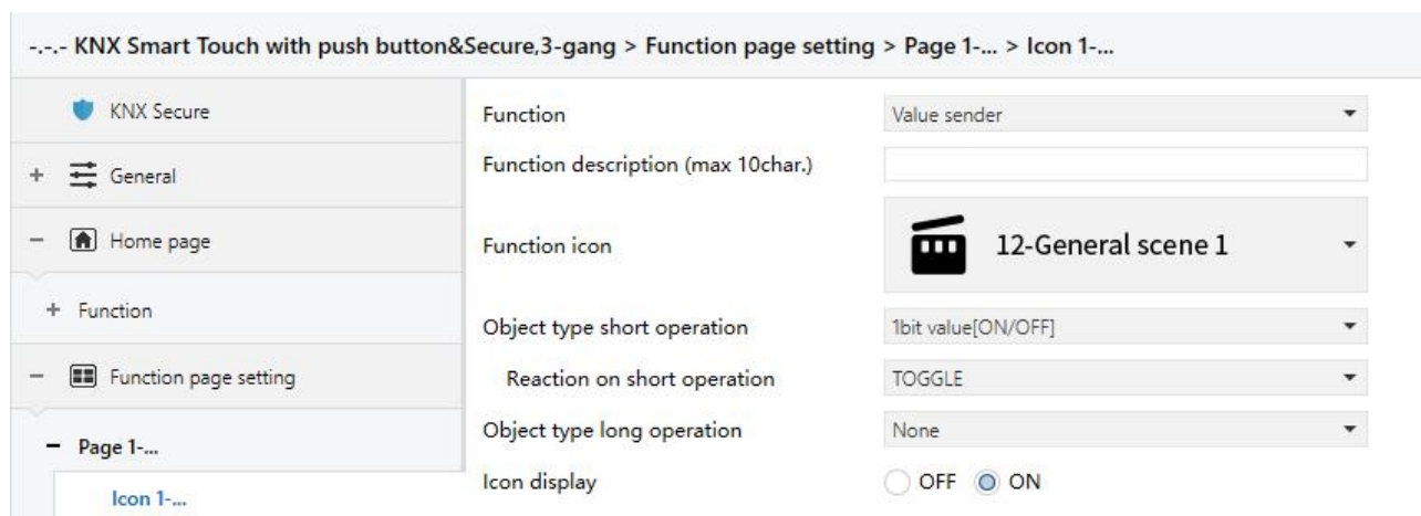
Fig.5.7.2.1 (6) Parameter setting of value sender
