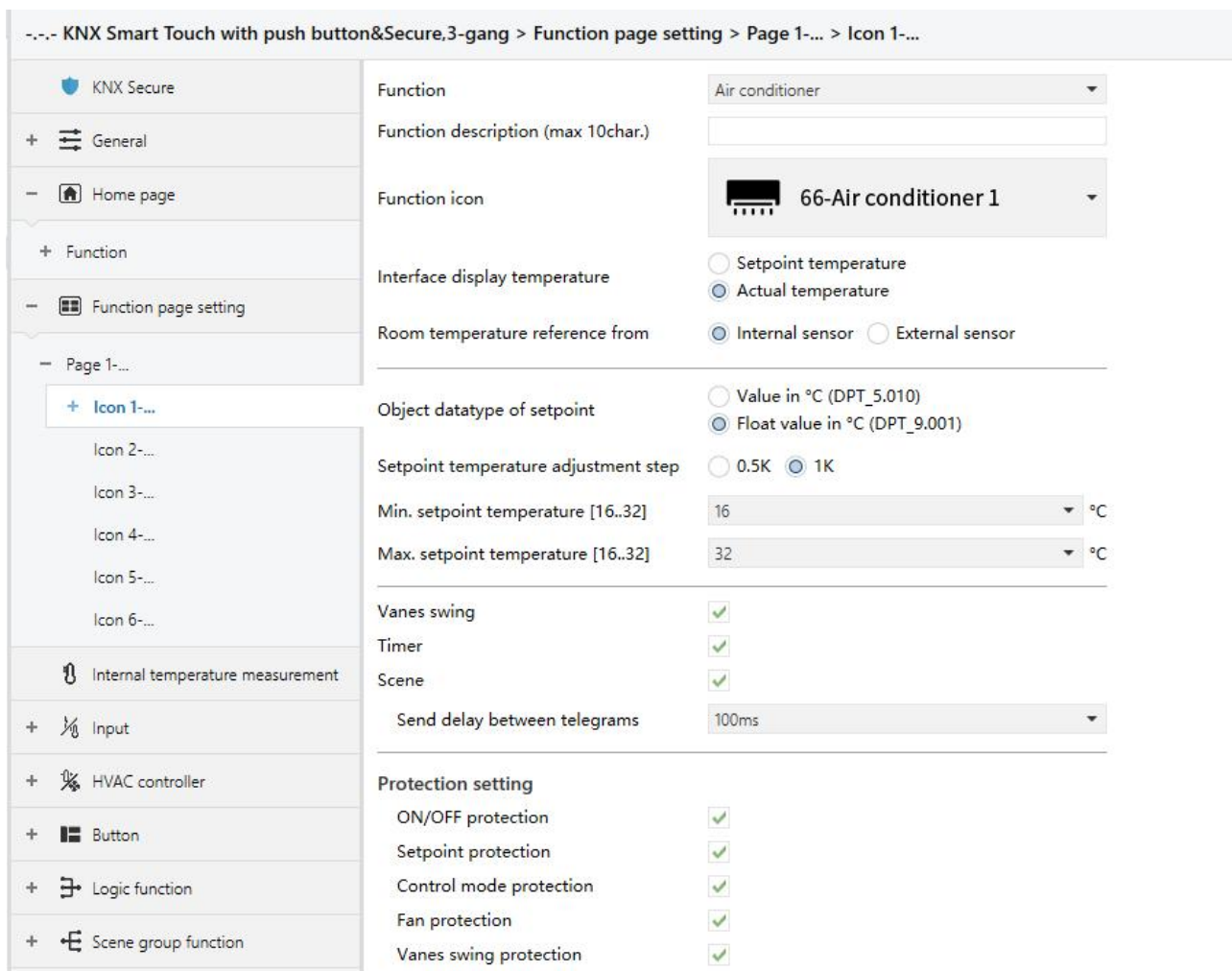
Fig.5.7.2.2(1) Air condition parameter window
