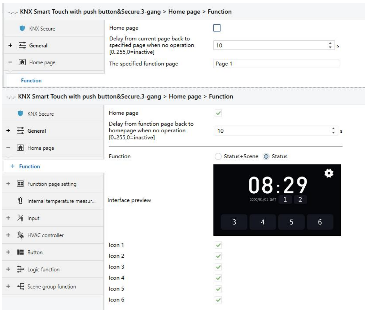
Fig.5.6.1 “Function” parameter window
