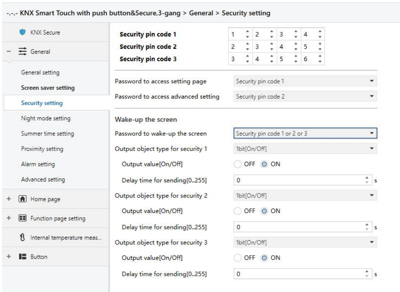
Fig.5.2.3 "Security setting" parameter window
