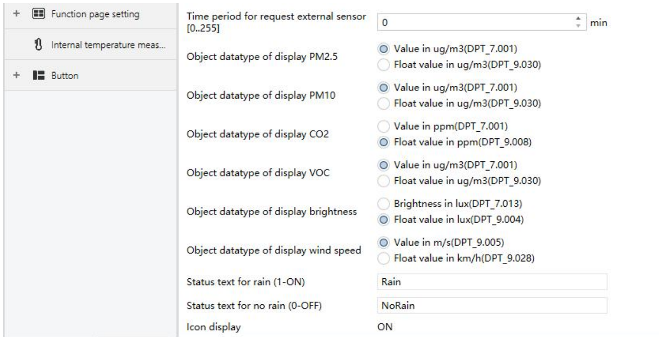
Fig.5.2.2 "Screen saver setting" parameter window
