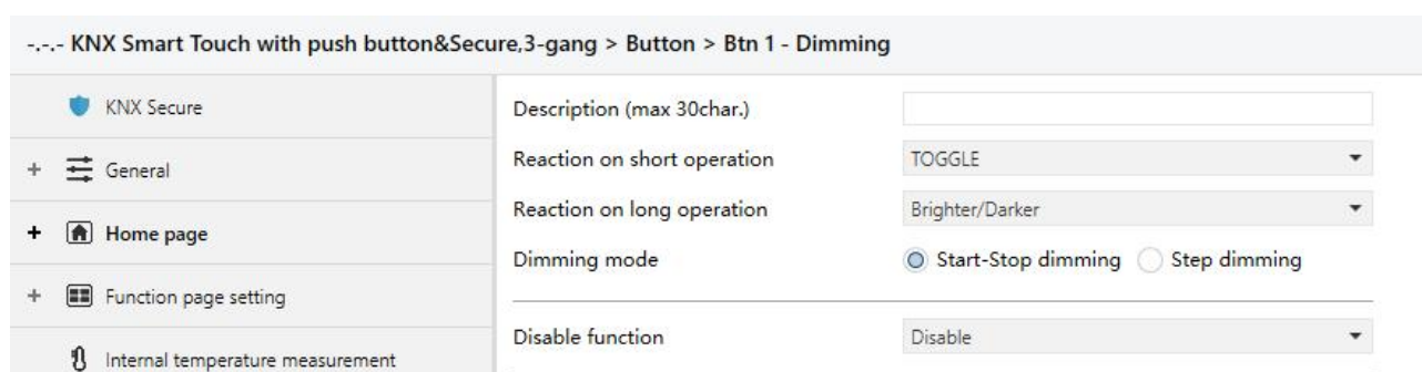
Fig.5.8.1.2 Parameter setting of dimming function
