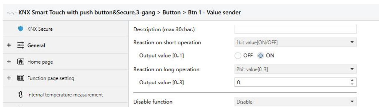
Fig.5.8.1.3 Parameter setting of value sender
