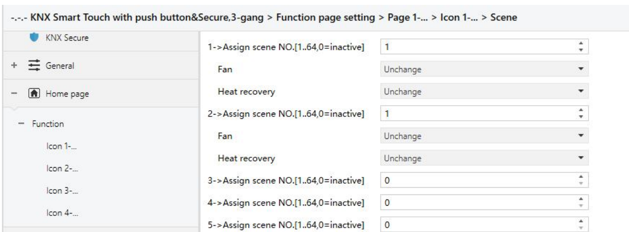
Fig.5.7.2.4(2) Ventilation system-scene parameter window
