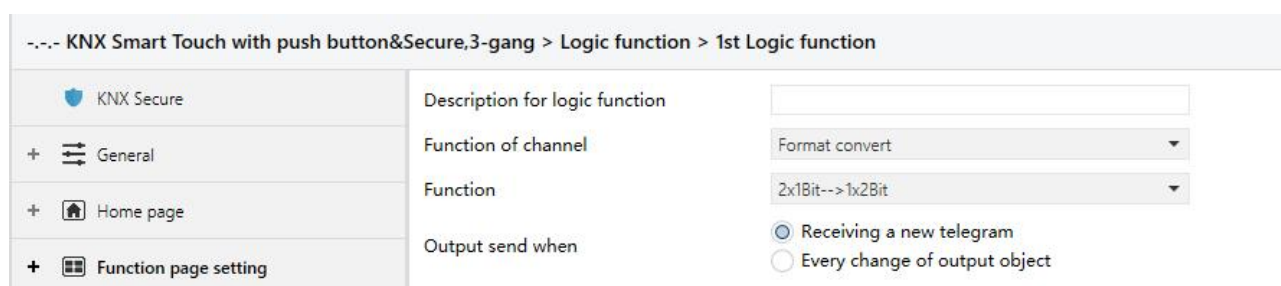
Fig.5.9.4 "Format convert" parameter window
