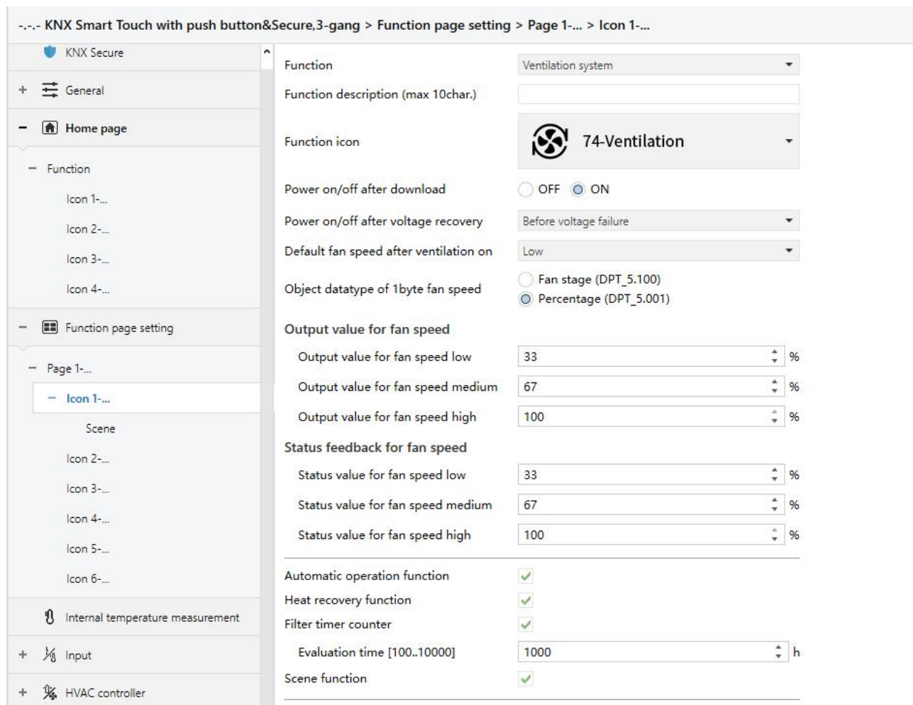
Fig.5.7.2.4 Ventilation system function parameter window
