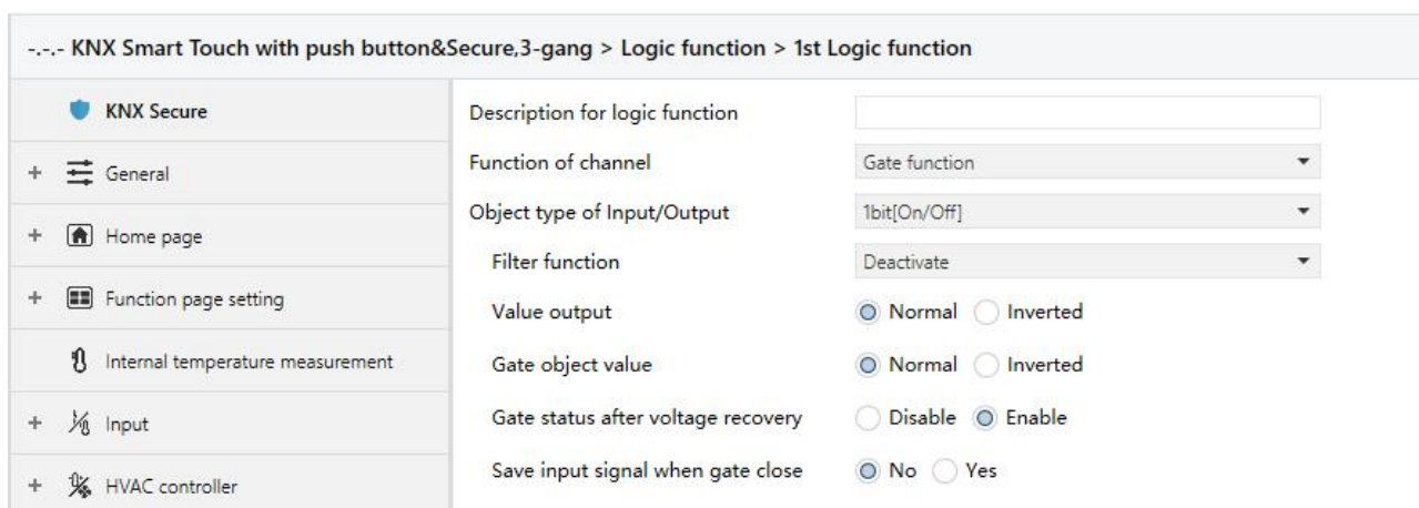
Fig.5.9.5 "Gate function" parameter window
