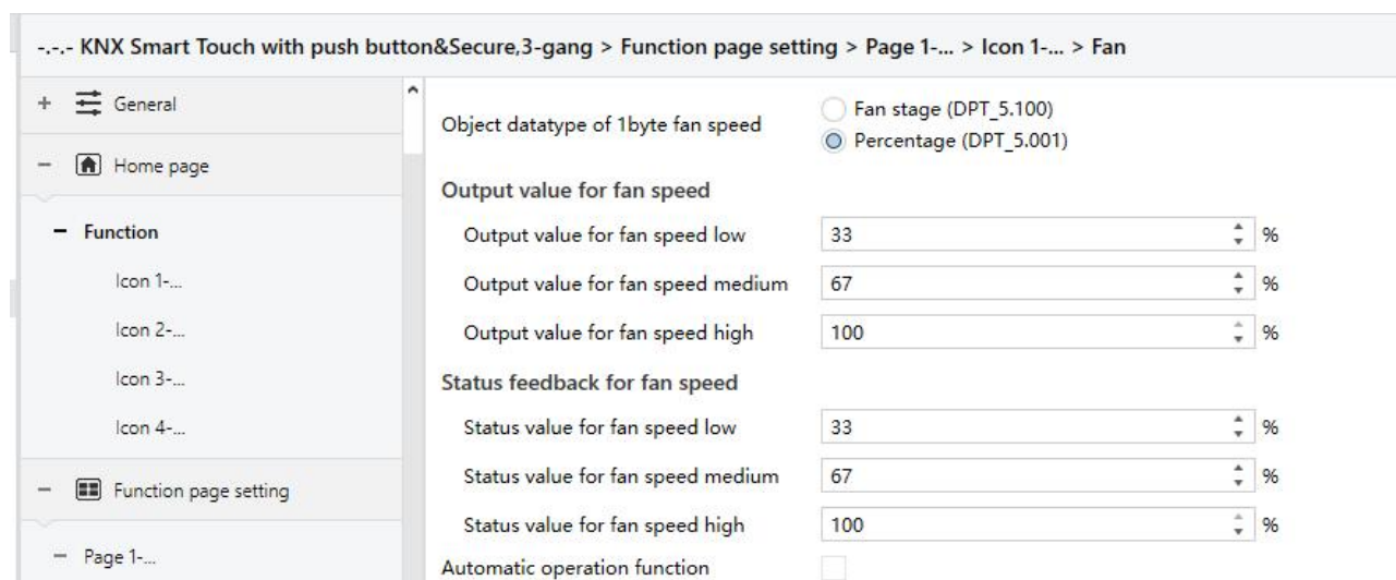
Fig.5.7.2.3(2) RTC -Fan speed parameter window
