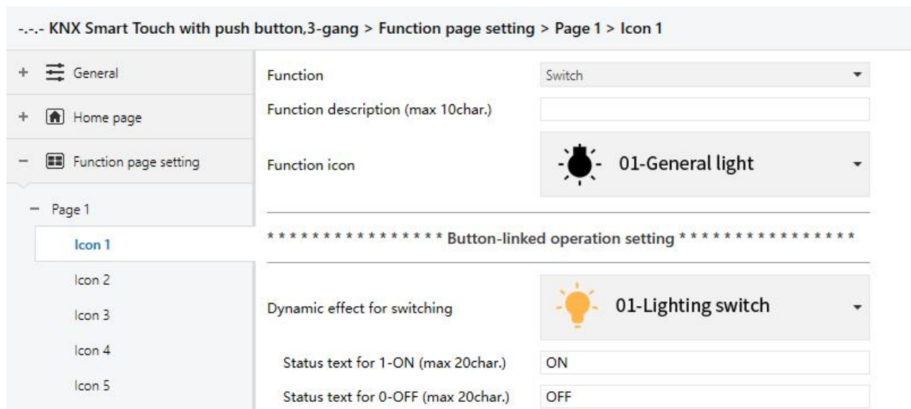
Fig.5.7.2.1 (1) Parameter setting of switch function
