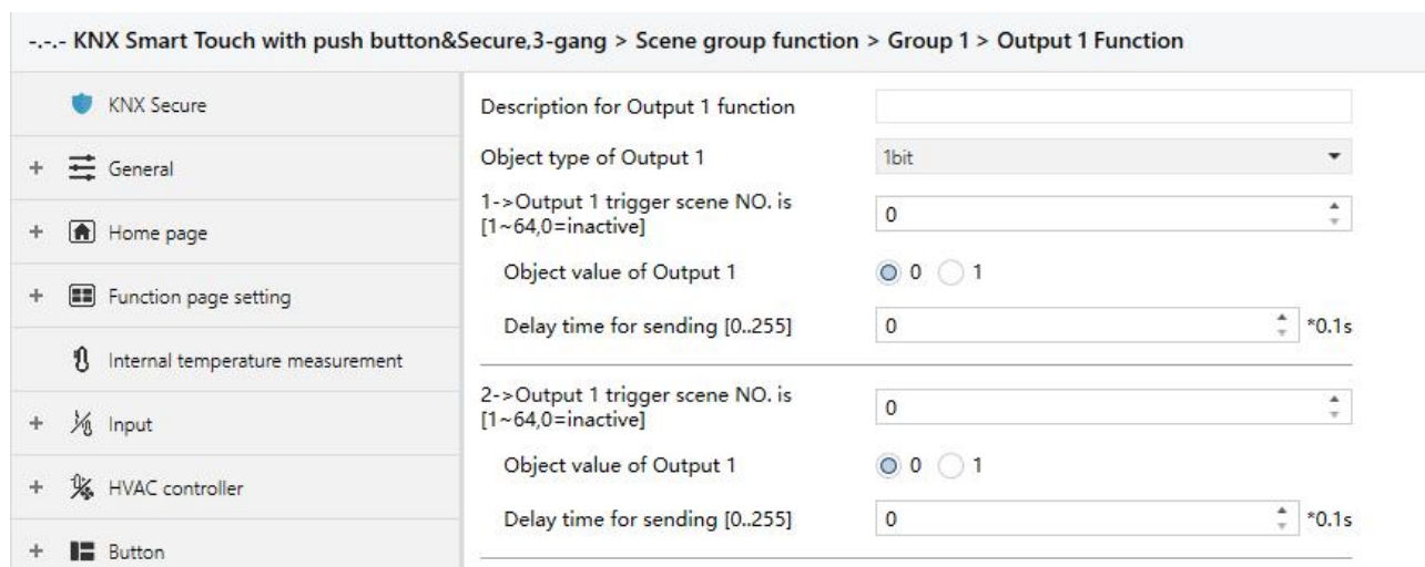
Fig.5.10 "Scene Group" parameter window
