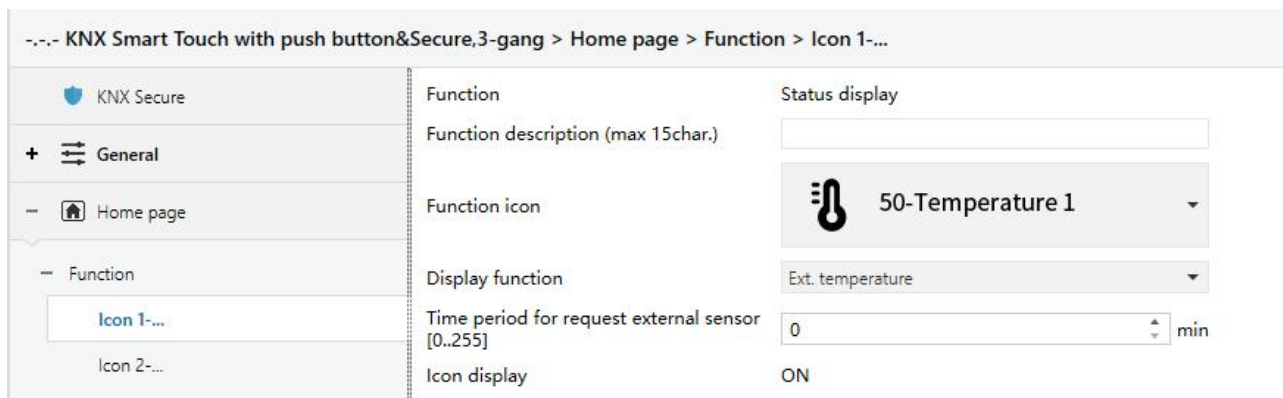
Parameter setting of status display
