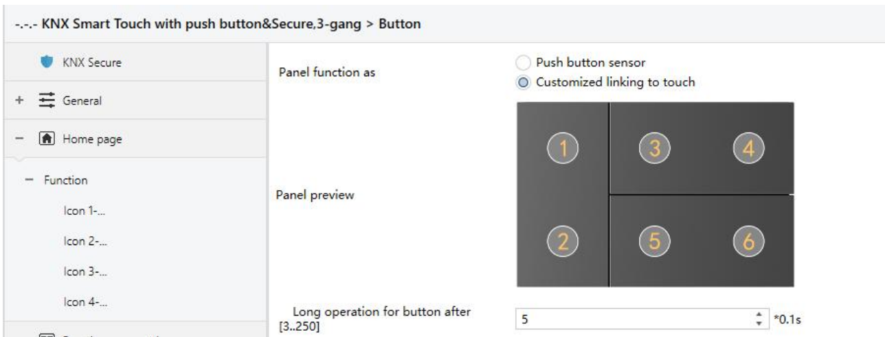
Fig.5.8 “Button” parameter window
