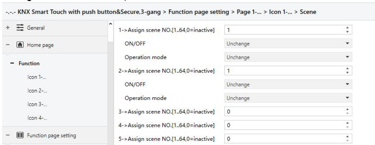
Fig.5.7.2.3(3) RTC-Scene parameter window
