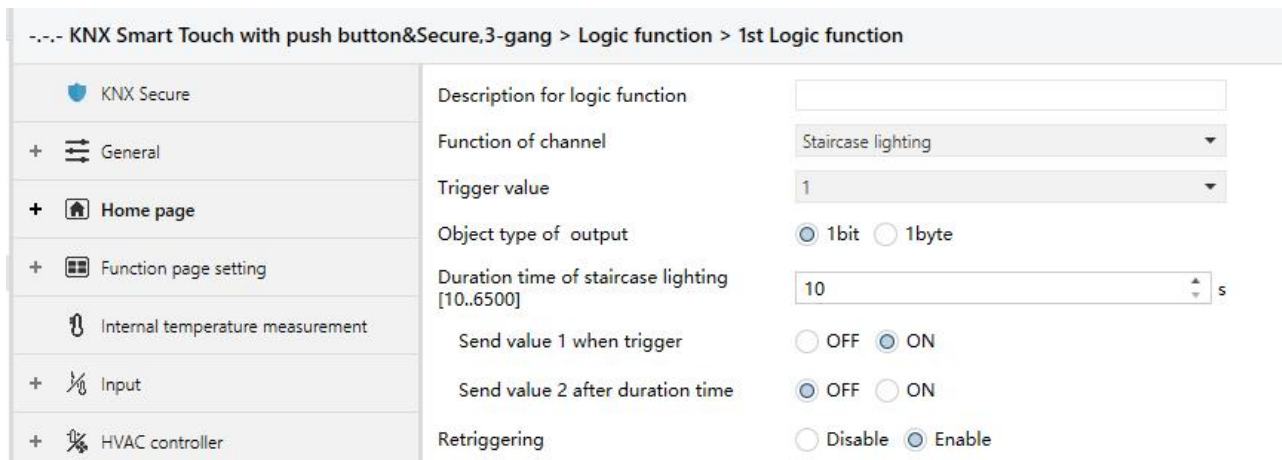
Fig.5.9.7 “Staircase lighting” parameter window
