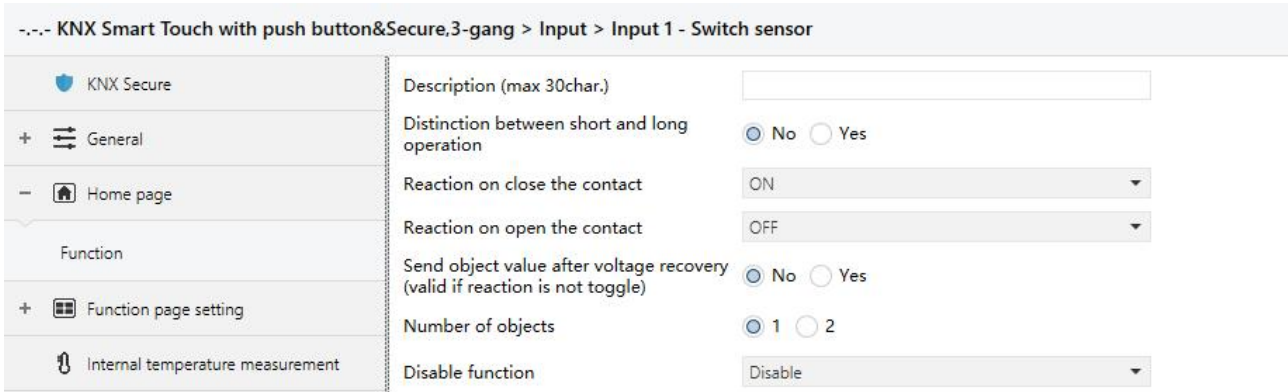
Fig.5.4.2(1) Parameter setting of switch sensor
