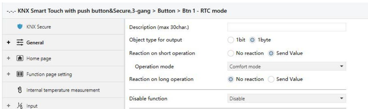
Fig.5.8.1.9 Parameter setting of RTC mode function
