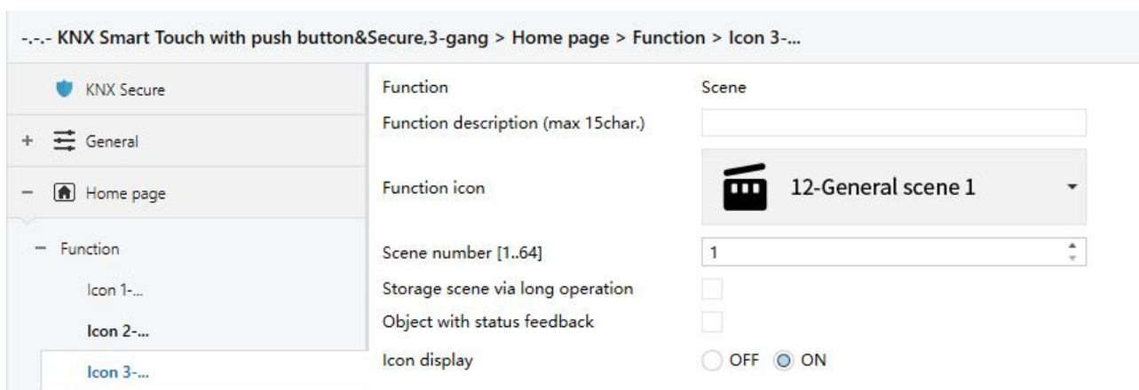
Parameter setting of scene function Fig.5.6.2 “Icon x” parameter window
