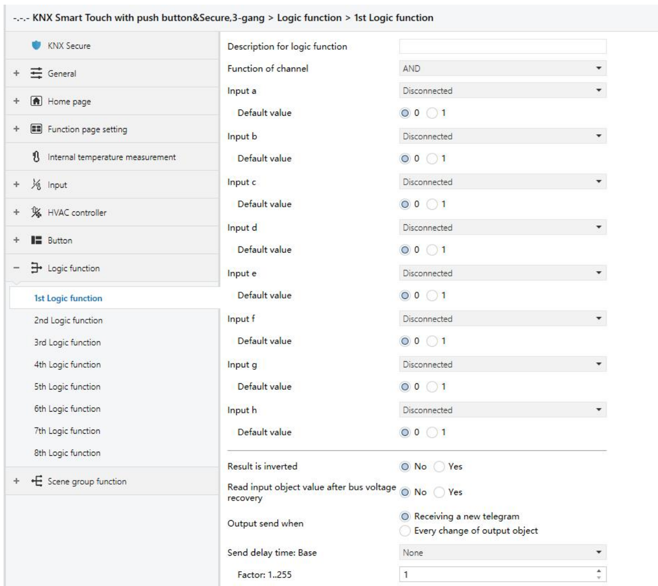
Fig.5.9.1 “AND/OR/XOR” parameter window
