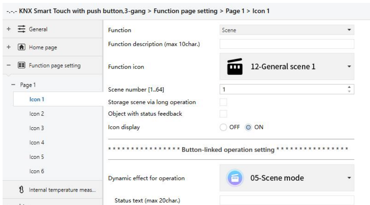
Fig.5.7.2.1 (7) Parameter setting of scene function
