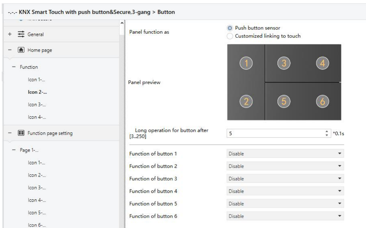
Fig.5.8.1 Parameter setting of button function
