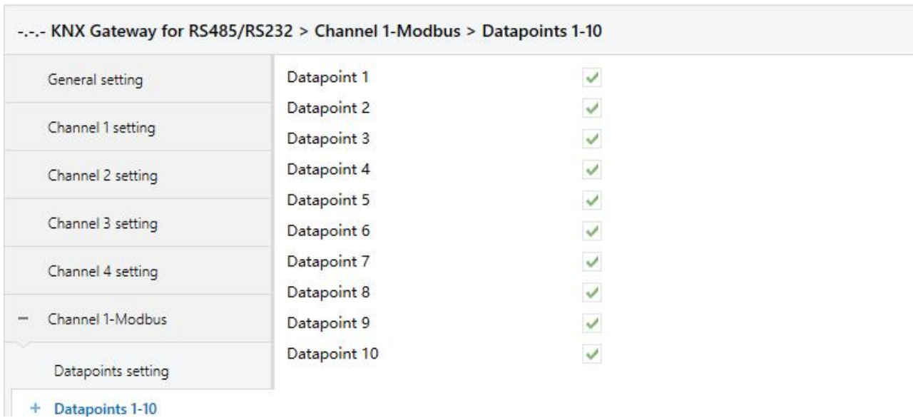
Fig.5.3.2.1 “Datapoints 1-10” parameter window
