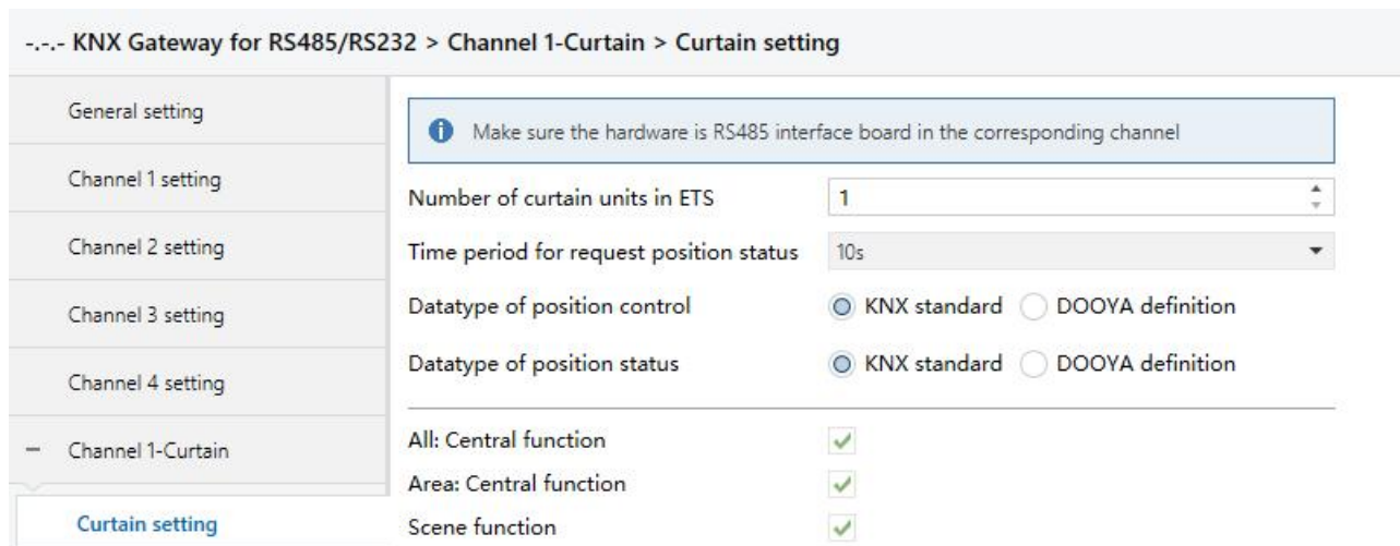
Fig.5.6.1 “Curtain gateway” parameter window
