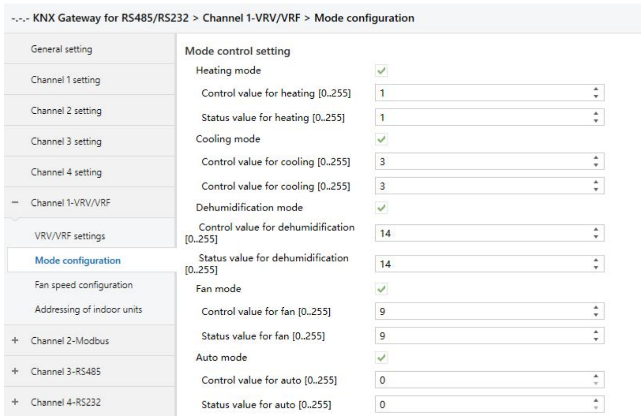
Fig.5.5.2 “Mode configuration” parameter window
