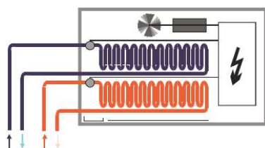
4-pipe fan coil
