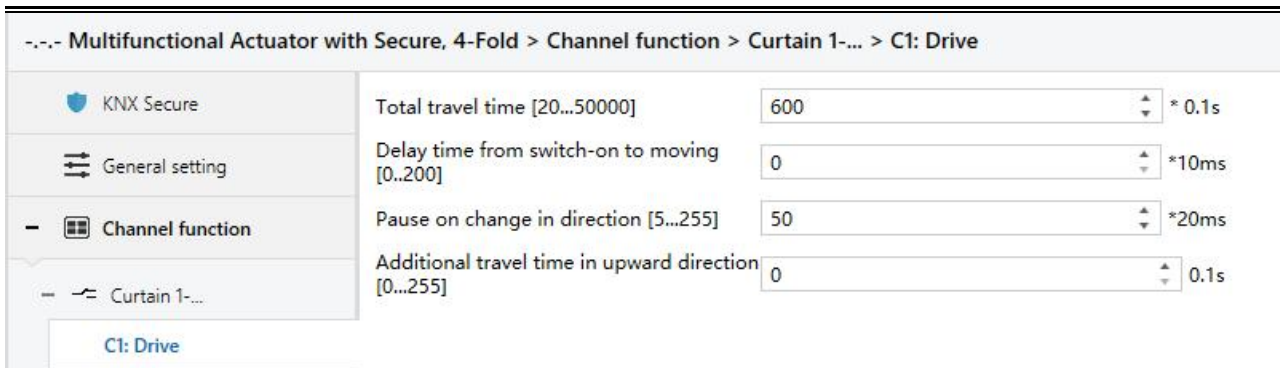
Fig. 4.6.1.1 Parameter window "Cx: Drive"
