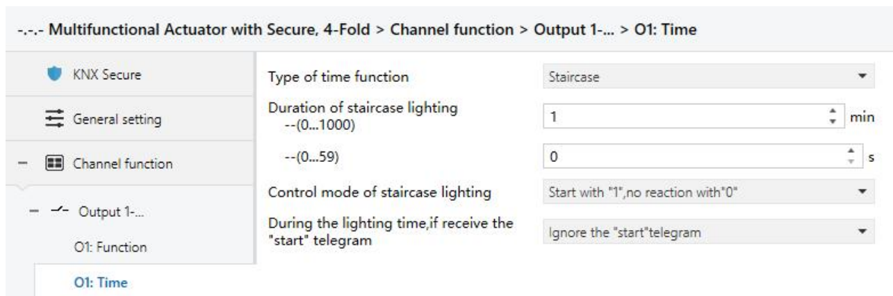
Fig. 4.4.2.3 Parameter window "Ox: Time-Staircase"
