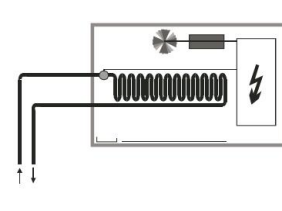
2-pipe fan coil
