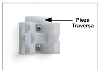
Fig. 4 Montaje en pared: lado plano hacia la pared, la pieza travesera semicircular hacia arriba.
