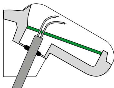
Fig. 11 Coloque el revestimiento del cable por debajo de la placa de circuitos impresos y conduzca solo los cables de conexión por las aberturas en la placa hacia arriba.
