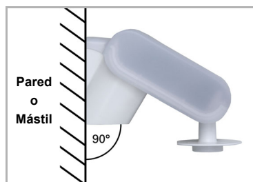
Fig. 2 El sensor de viento/lluvia debe montar en una pared vertical (o poste).
