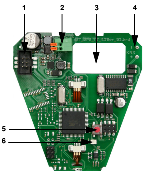
Fig. 13 1) Conexión por cable al sensor de precipitación en la tapa de la caja 2) Clema de conexión rápida para la fuente de alimentación (20...30 V DC), Cable rígido de hasta 1,5 mm 2 o flexible. Ocupación de bornes independiente de la polaridad (+/- o -/+) 3) Apertura para el cable de la fuente de alimentación, el cable de Bus 4) Conexión por clema de Bus KNX +/- 5) Botón de programación 6) LED de programación
