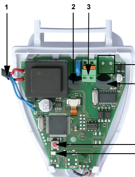
Fig. 12 1) Conexión de cable al sensor de lluvia en la cubierta del gabinete 2) Abertura para cables de alimentación 3) Terminal de resorte de alimentación (230 V AC), apto para conductores sólidos de hasta 1,5 mm 2 o conductores de hilo fino 4) Ranura para terminal KNX +/- 5) Orificios para el cableado de bus 6) Tecla de programación para sincronizar el dispositivo 7) LED de programación
