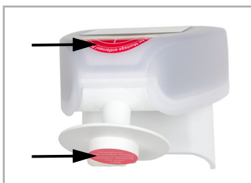
Fig. 17 Después de la instalación, retire la etiqueta protectora del sensor de viento y la etiqueta de información de "Distancia" en la parte superior de la cubierta.
