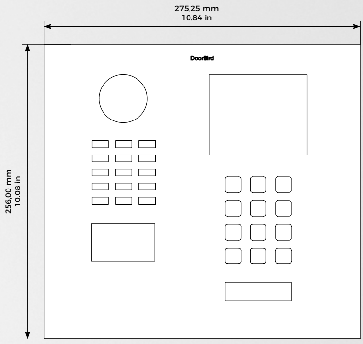
Placa frontal
